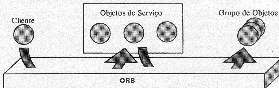
Figura 2.2 - Execução de uma requisição na abordagem de serviço
