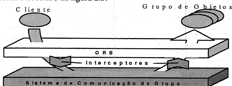
Figura 2.3 - Execução de uma requisição na abordagem de interceptação
