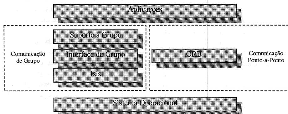
Figura 3.1 – Estrutura da implementação da abordagem de serviço
