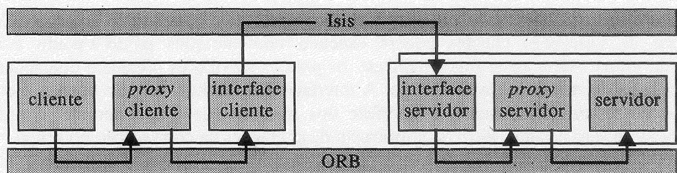
Figura 3.2 – Difusão de mensagem na implementação da abordagem de serviço
