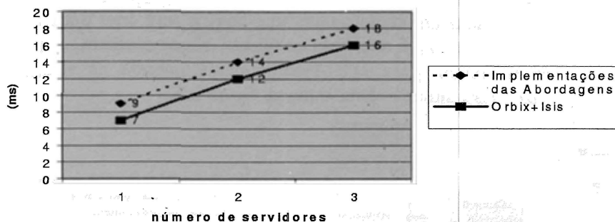
Figura 3.6 – Tempo médio de resposta de acordo com o número de servidores
