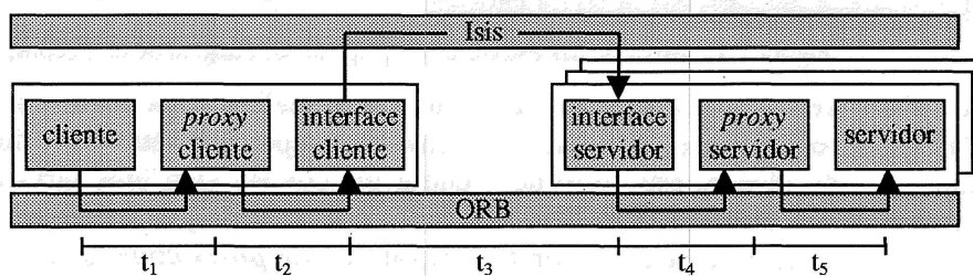
Figura 3.7 – Tempos de resposta parciais nas implementações desenvolvidas
